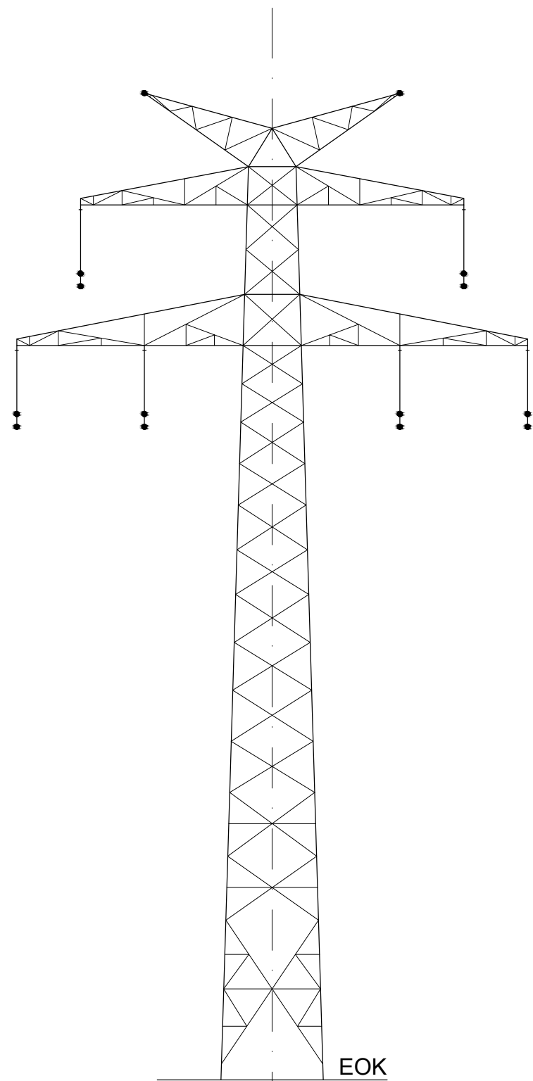
Donaumast geteilte Erdseilspitze
