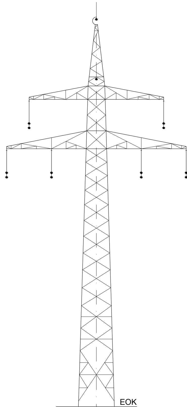
Donaumast einfache Erdseilspitze
