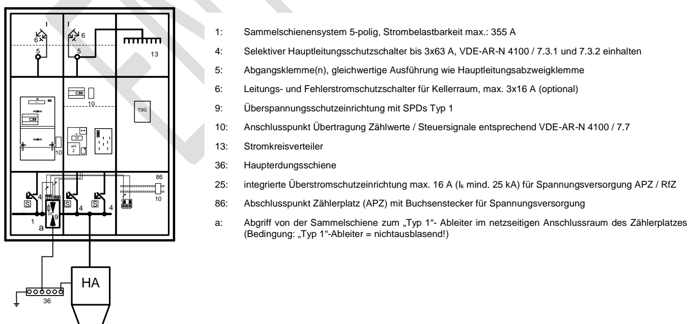
Abb. 1: Spannungsversorgung aus SPD Typ 1
